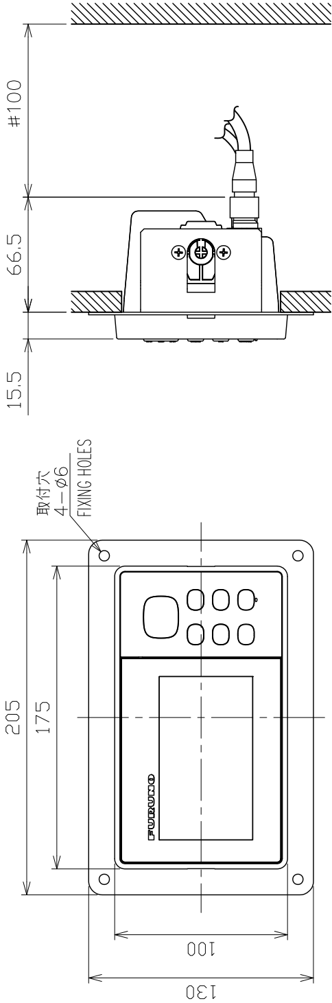
4-取付穴位置 PILOT HOLES
