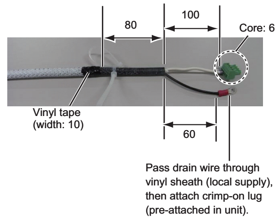
TTYCSLA-4 cable
