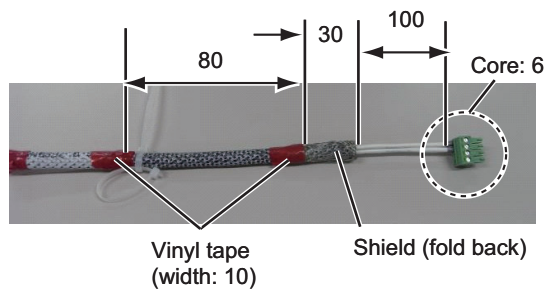
TTYCS-1 cable
